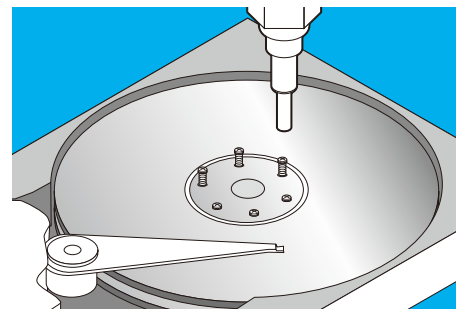
ブルーレイドライブ 薄型シャーシへの精密ねじ締め
