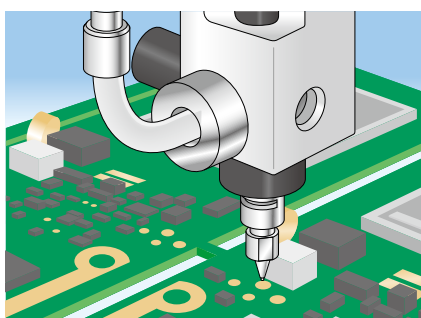
基板へのクリーム半田塗布
